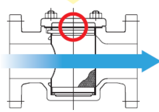
ストレート形ストレーナ 圧力損失小
